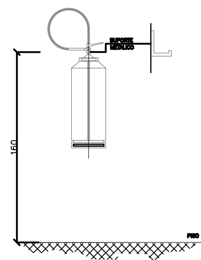
DETALHE 4 EXTINTORES - EM PAREDE SEM ESCALA
