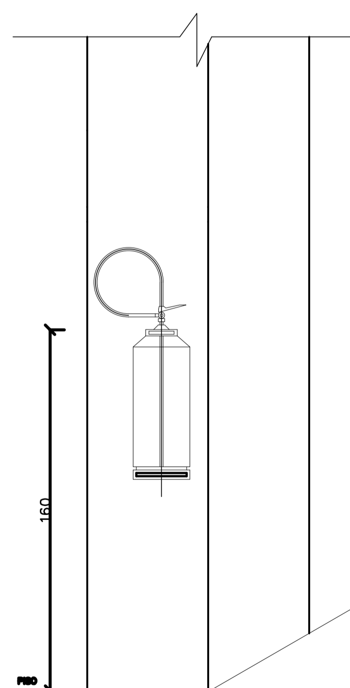
DETALHE 5 EXTINTORES - EM PILAR SEM ESCALA
