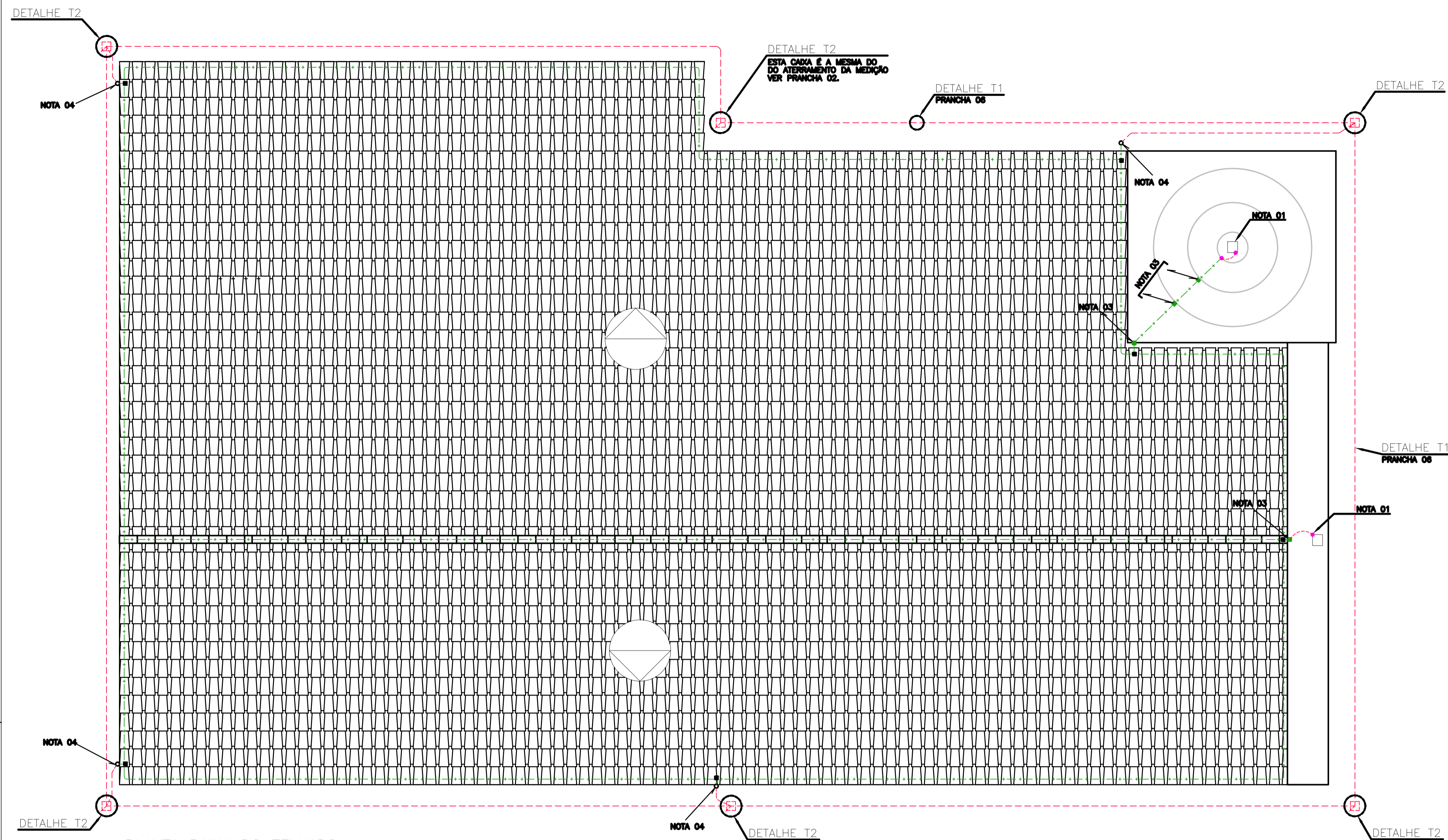
PLANTA BAIXA DO TELHADO ESCALA: 1/50
