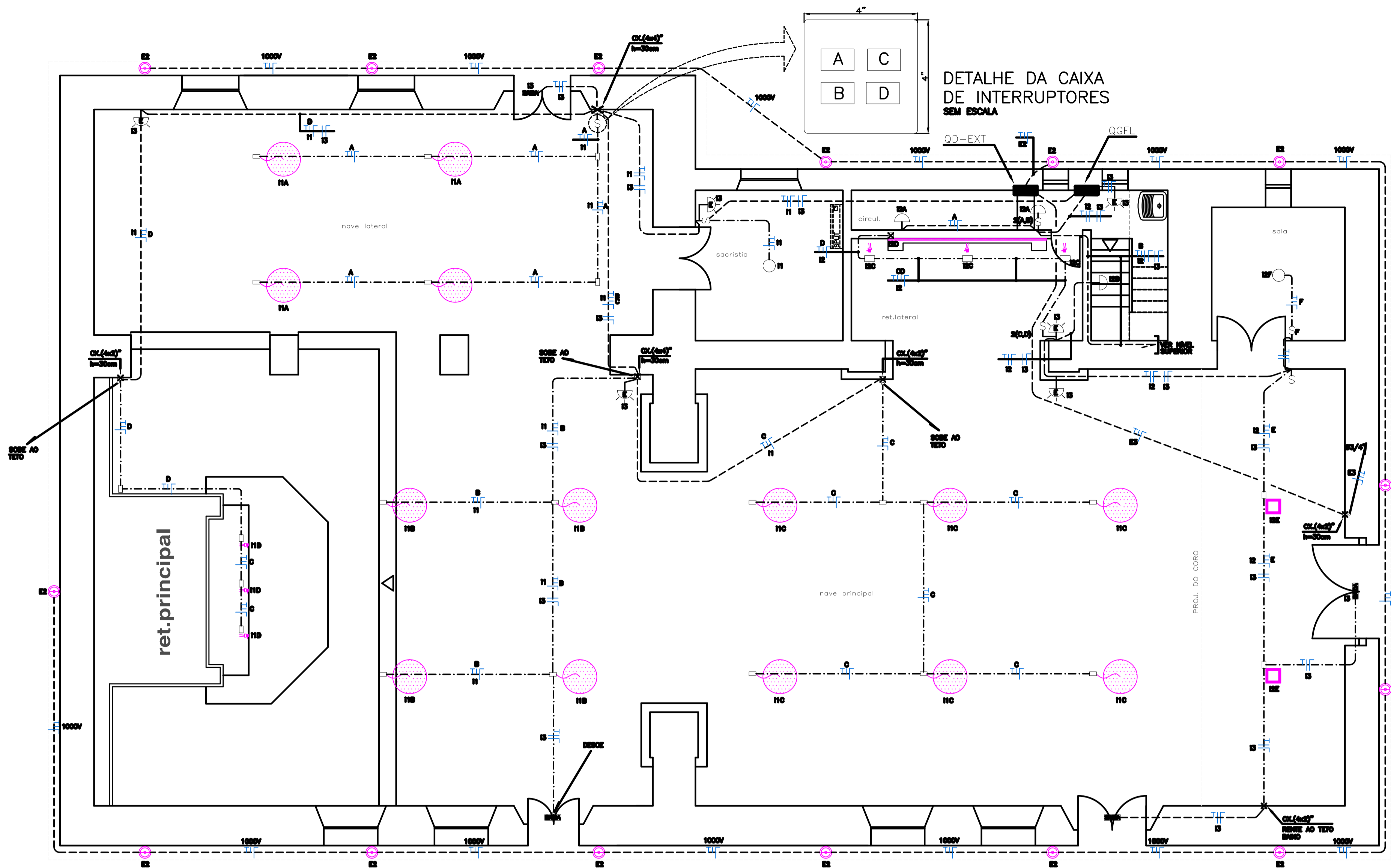
PLANTA BAIXA DO TÉRREO (ILLUMINAÇÃO) ESCALA: 1/50
